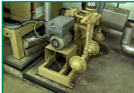
Modulerende aardgastoevoer en frequentieregelaar op de voedingswaterpomp
